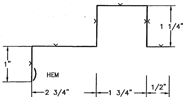
DOOR HAT TRIM
